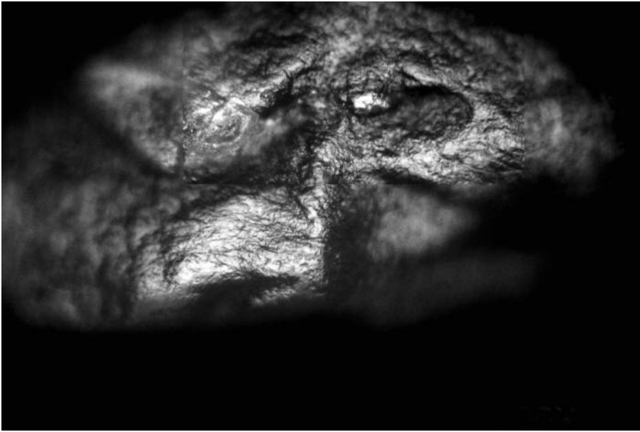
Fig. 4 - Politura dovuta a taglio di tessuti animali poco resistenti. Ingrandimento: 200x. - Cutting soft animal materials polish. Magnification: 200x.
