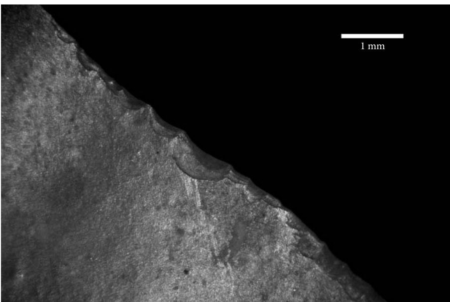
Fig. 6 - Sbrecciature attribuite a taglio di materiale poco resistente. - Cuttin soft material micro-scarring.
